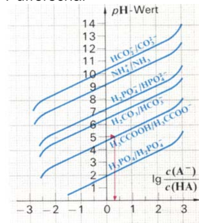
B 71.1. Pufferschar. Jedes der angeführten Puffersysteme hat für den Fall c(\text{Base})/(\text{Säure}) = 1 den pH-Wert, bei dem die Gerade die Ordinate schneidet. Der pH-Wert einer Pufferlösung mit c(\text{Base})/c(\text{Säure}) \neq 1 kann näherungsweise graphisch ermittelt werden (rote Pfeile).
